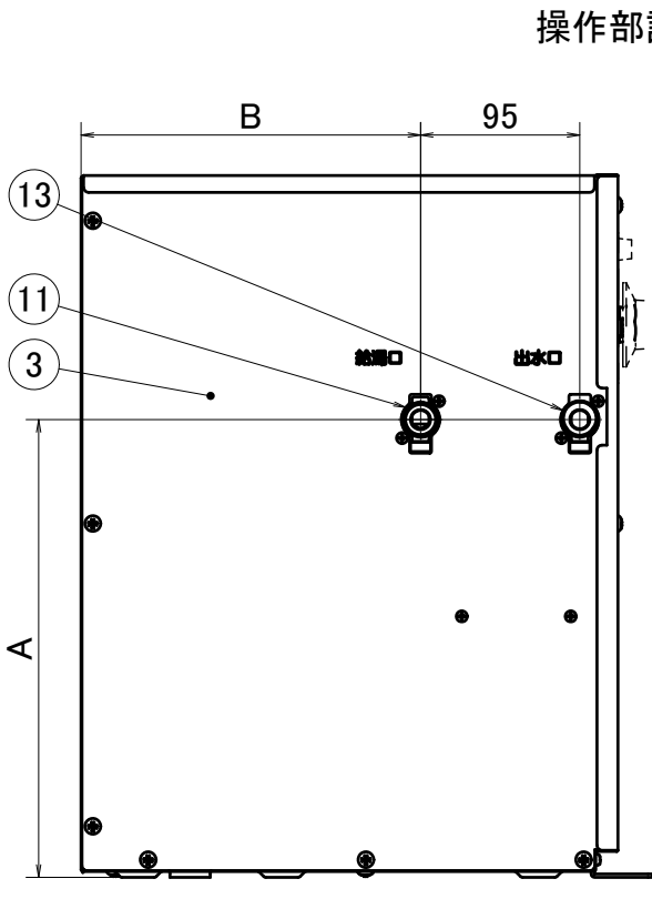
左側面図
