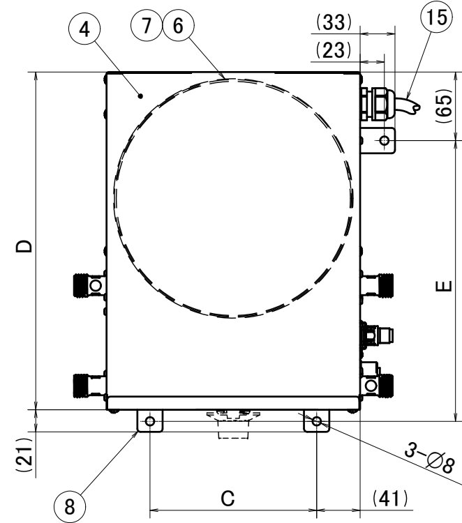
平面図
