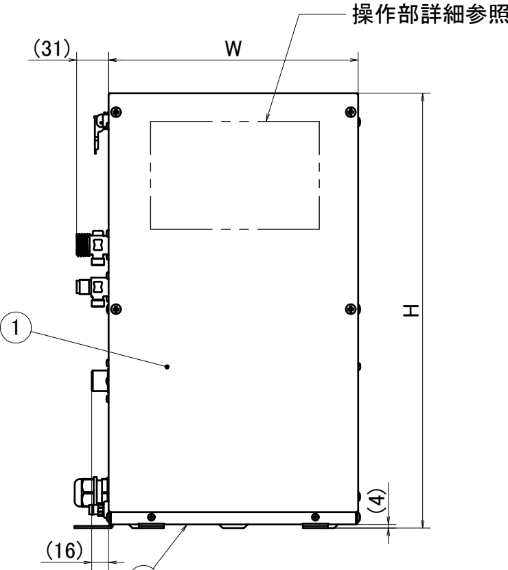
正面図
