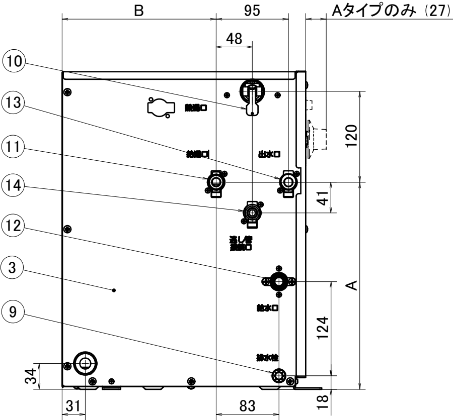
左側面図
