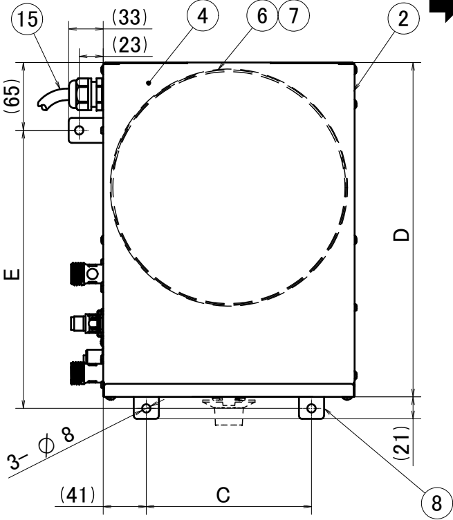
平面図
