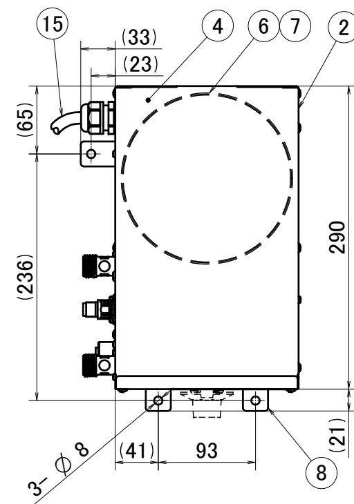
平面図
