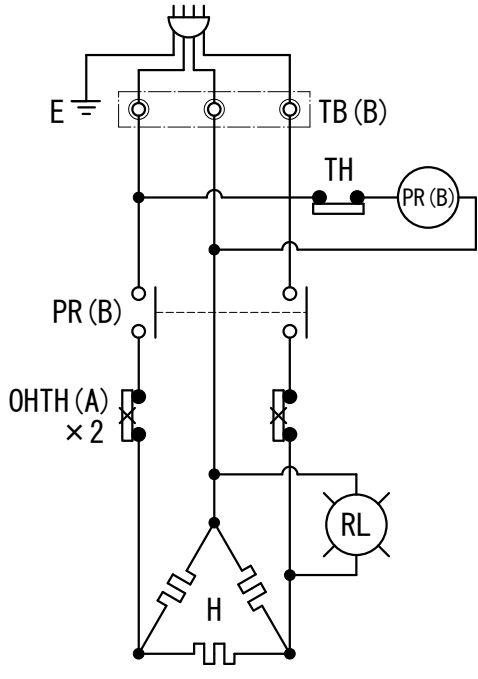
⑤ 三相
