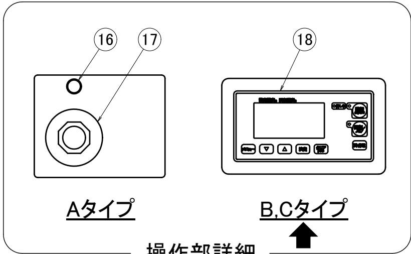
操作部詳細
