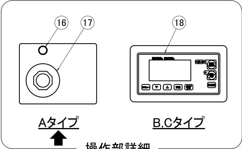
操作部詳細
