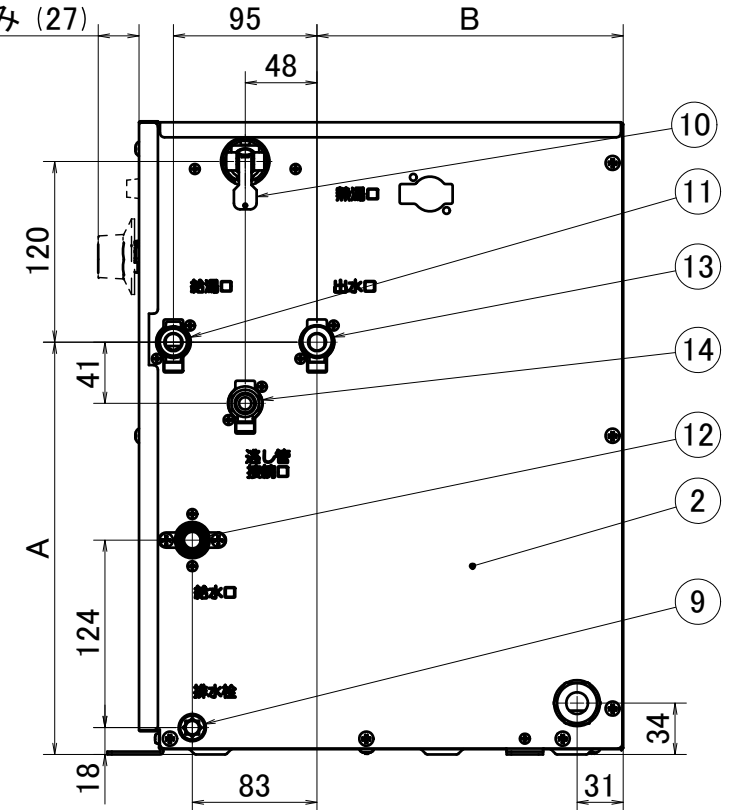
右側面図
