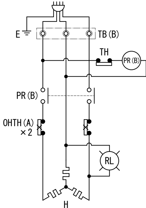
④ 三相
