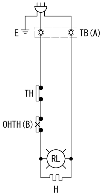
② 単相
