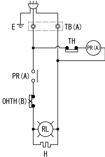
③ 単相
