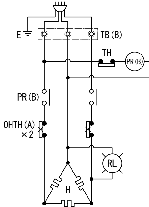
⑤ 三相
