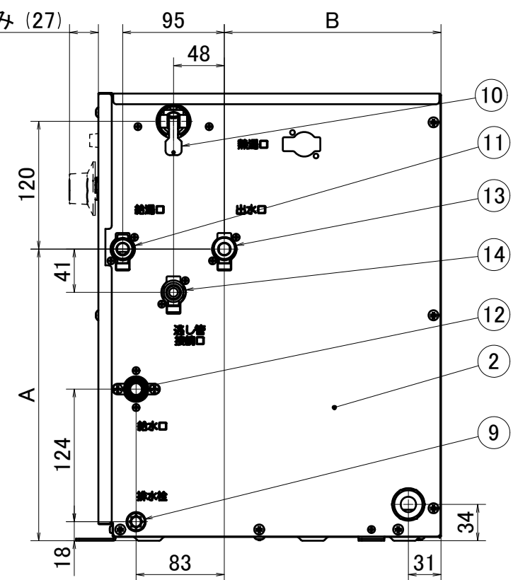
右側面図
