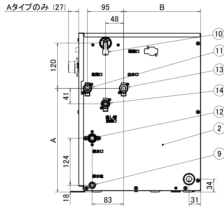
右側面図
