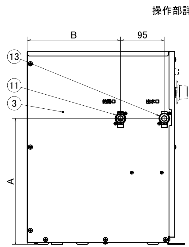
左側面図
