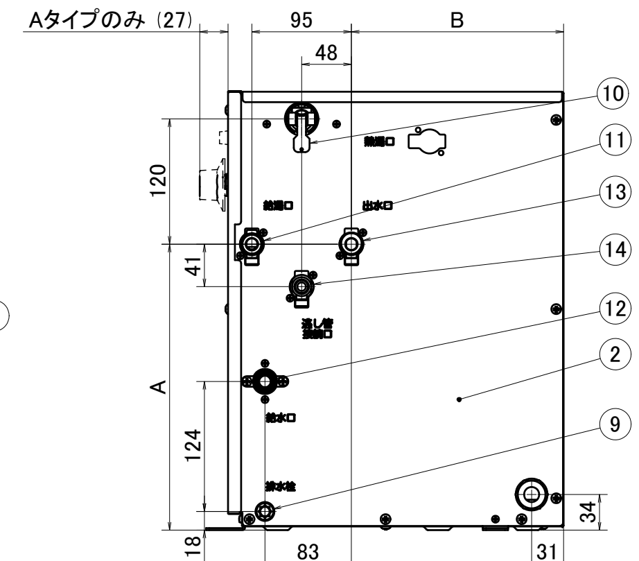
右側面図
