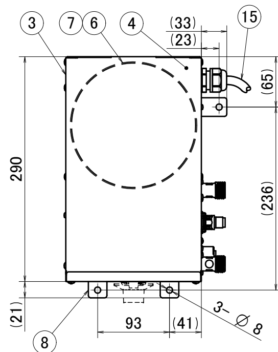
平面図
