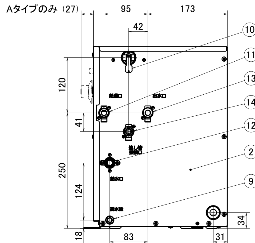
右側面図
