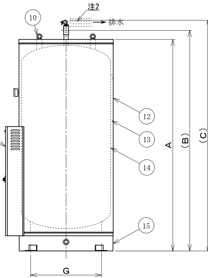
右側面図
