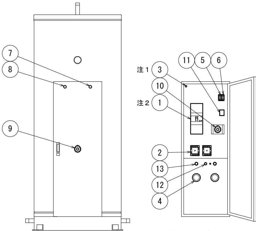
電装ケース部品配置図
