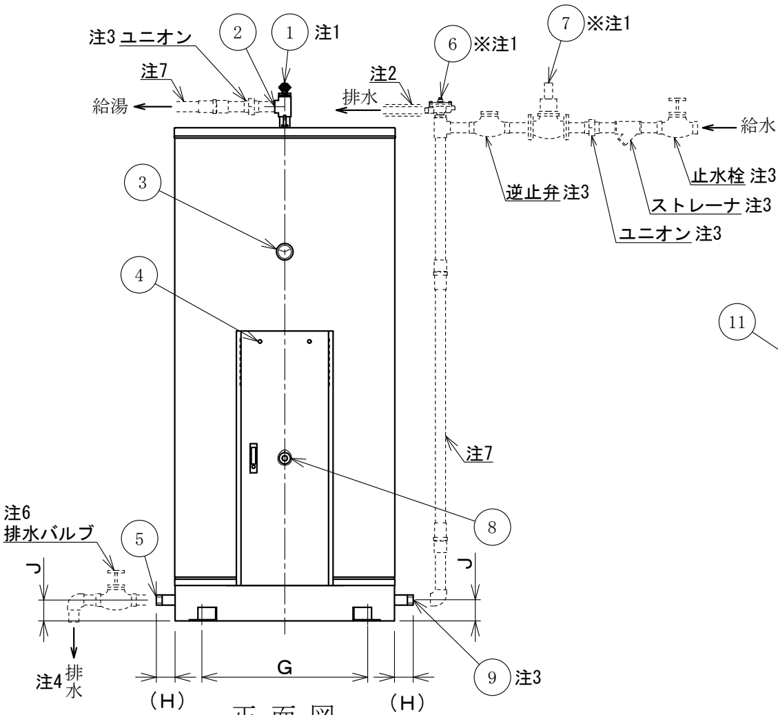
正面図
