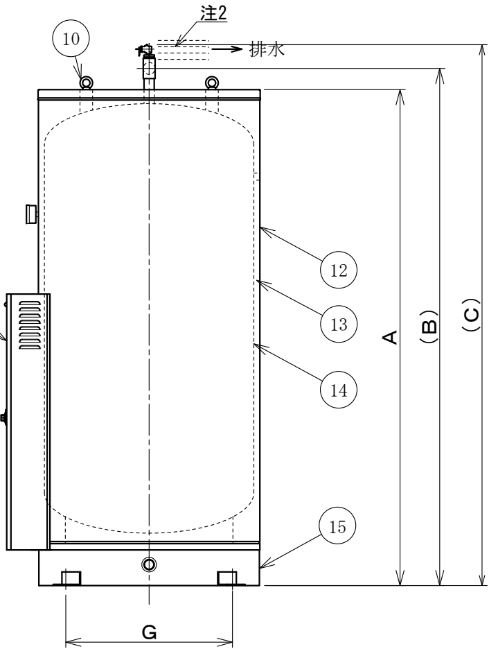
右側面図
