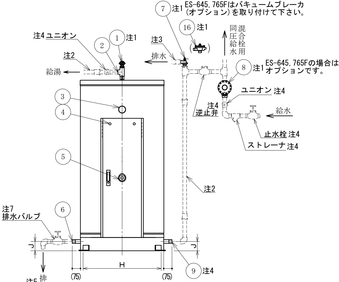
正面図
