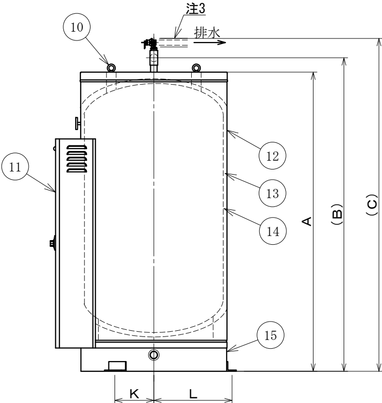
右側面図
