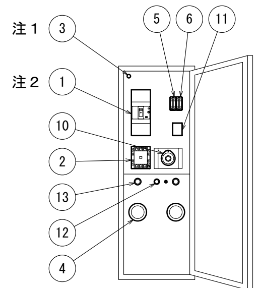
電装ケース部品配置図
