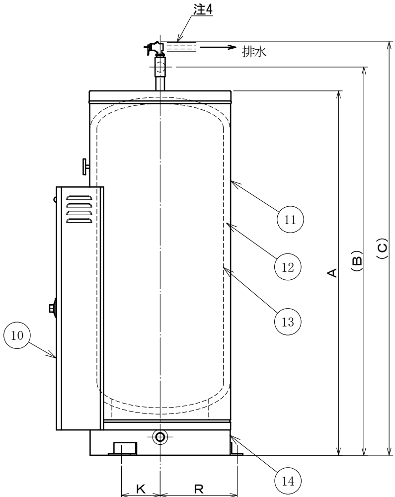
右側面図
