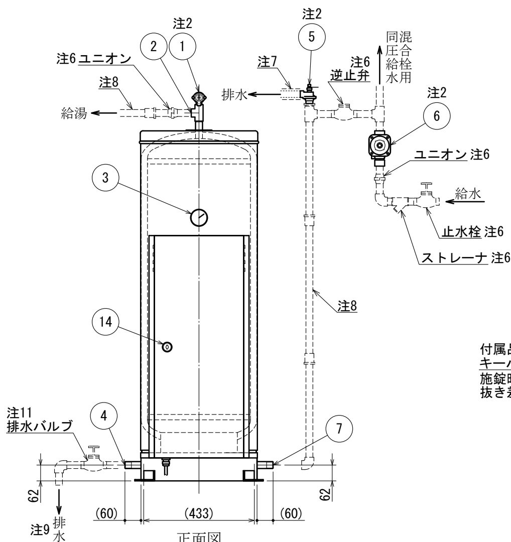
正面図
