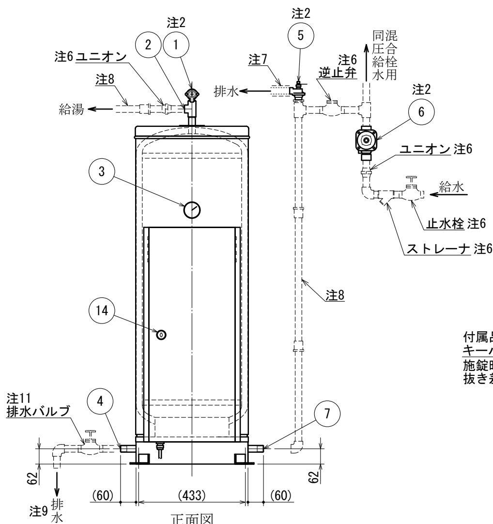
正面図
