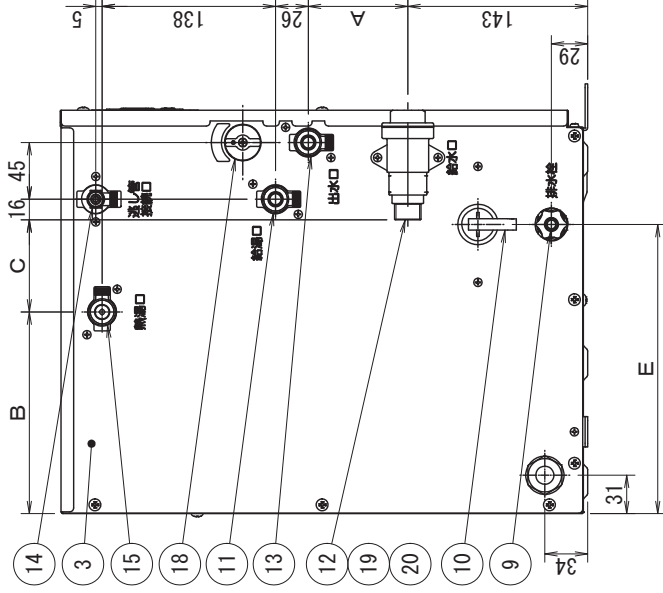
固定ねじ穴位置図
