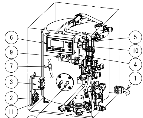
部品配置図 (図はESD20B/CRX)
