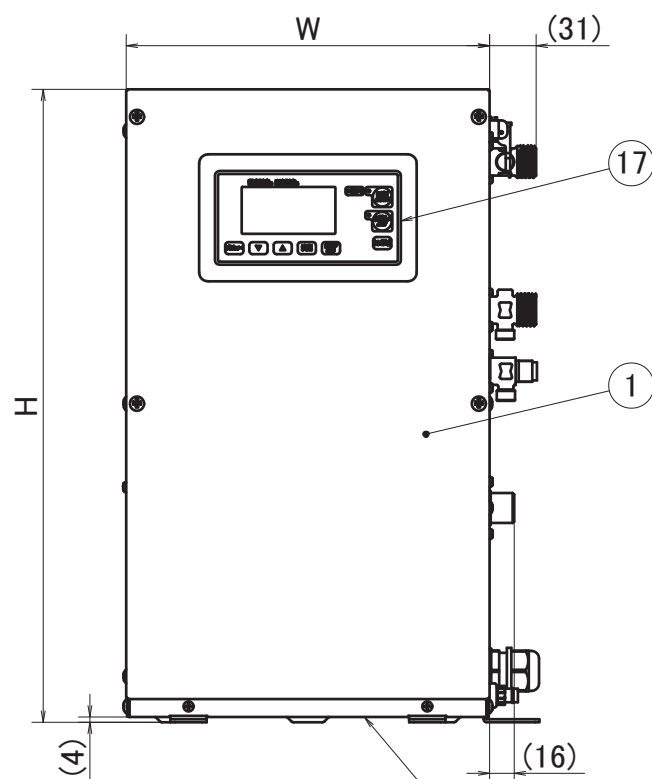
正面図
