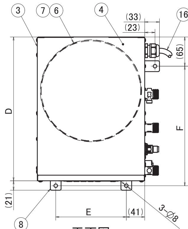
平面図
