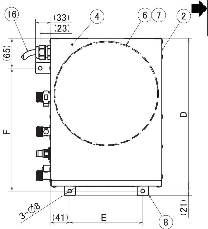
平面図
