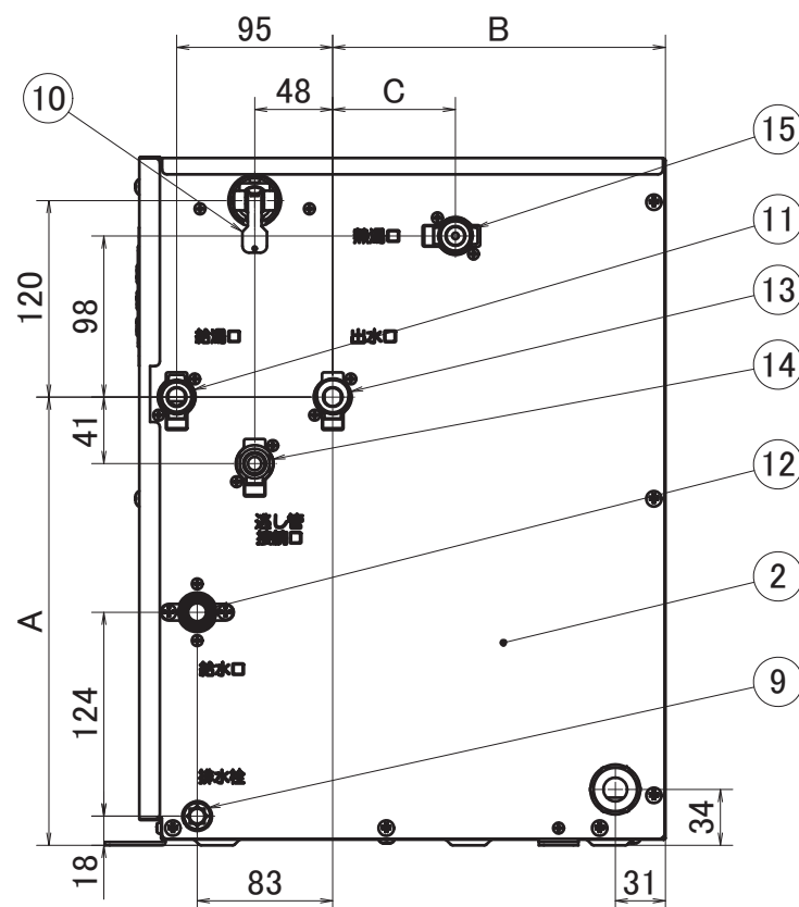
右側面図
