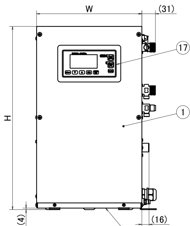
正面図
