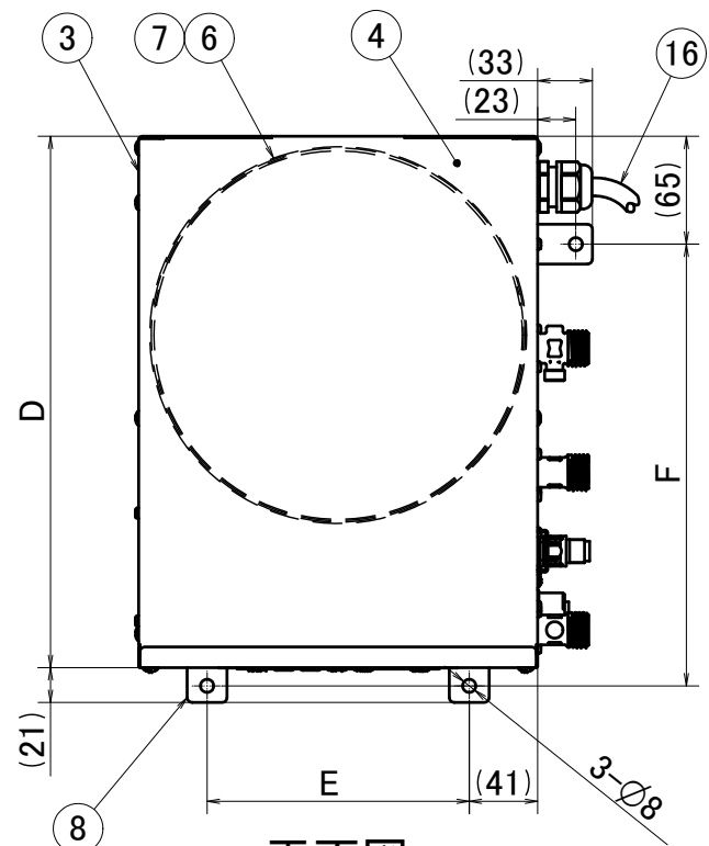
平面図
