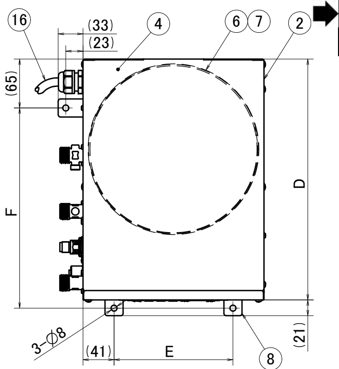
平面図
