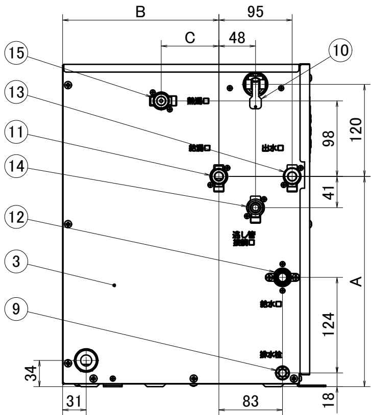
左側面図
