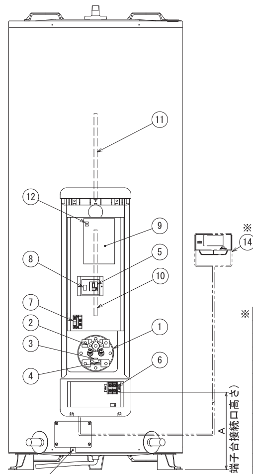
注2 部品配置図
