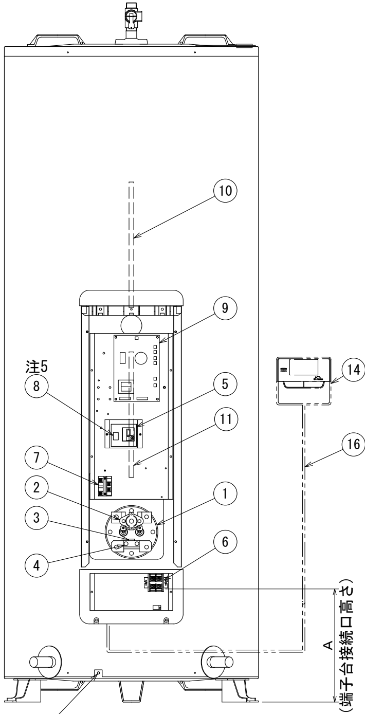
部品配置図
