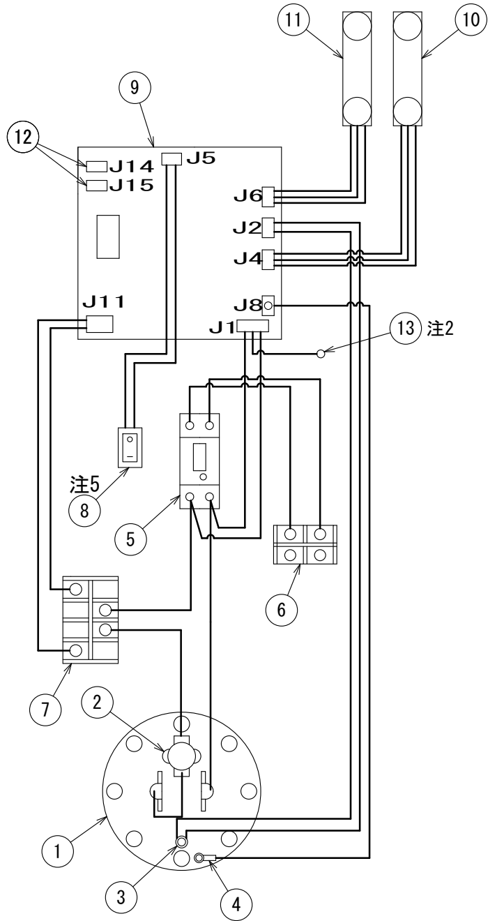
配線図
