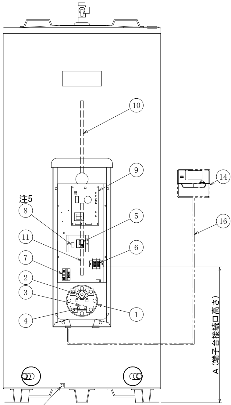
部品配置図
