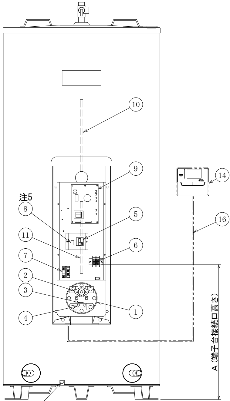
部品配置図
