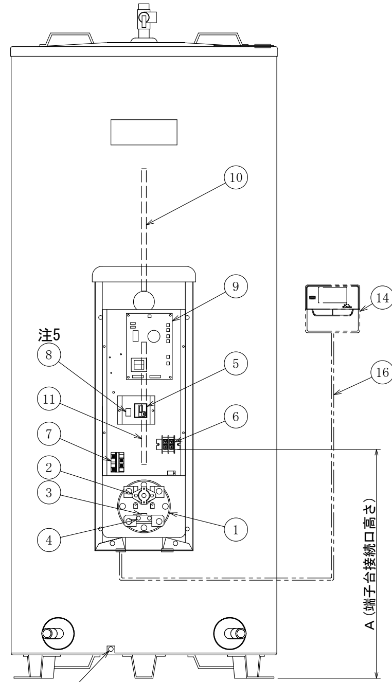
部品配置図
