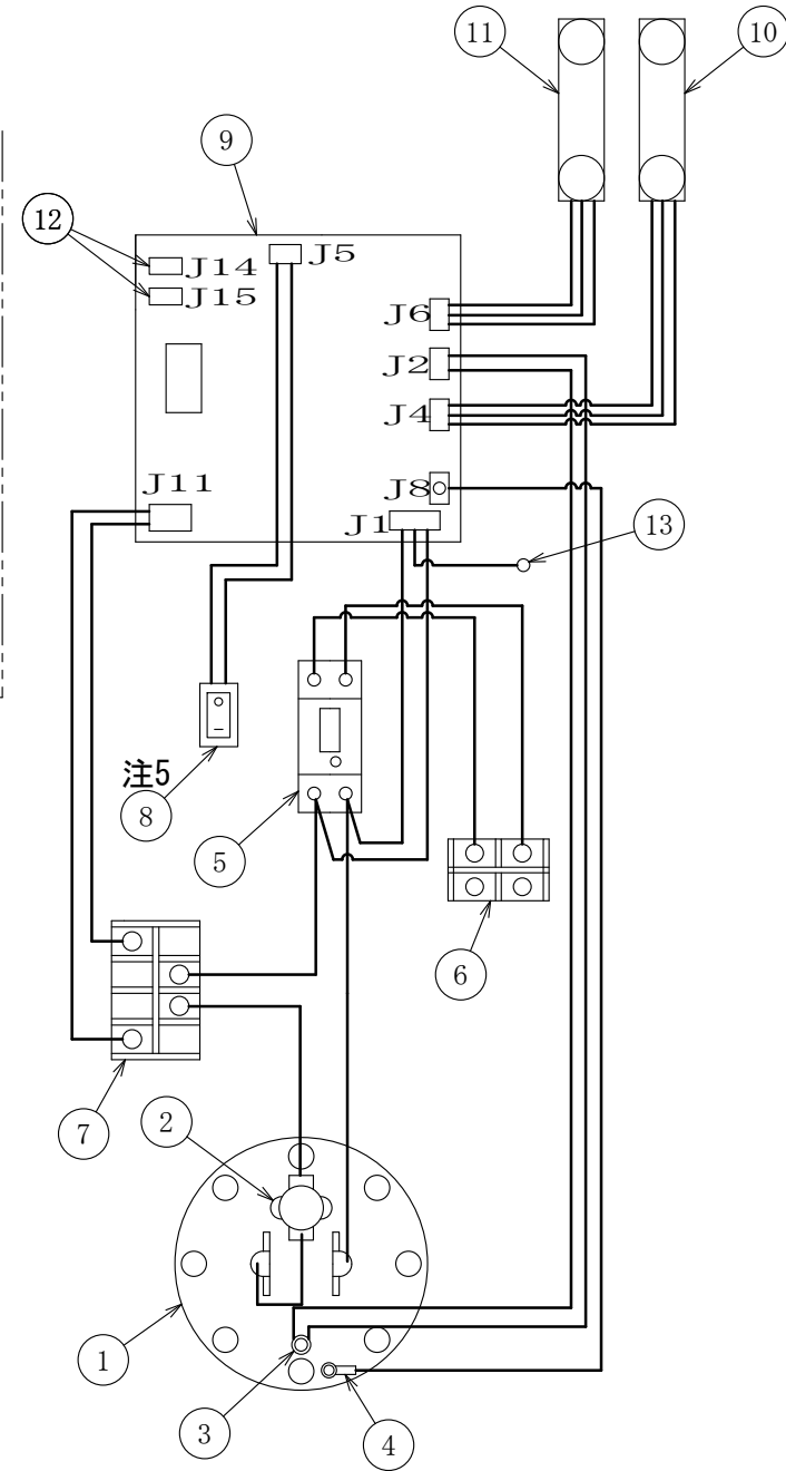
配線図
