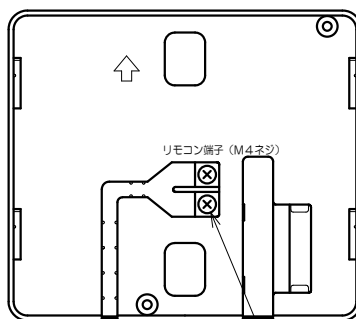
背面図
