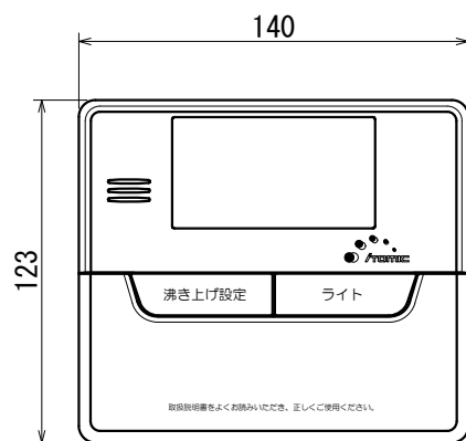
正面図
