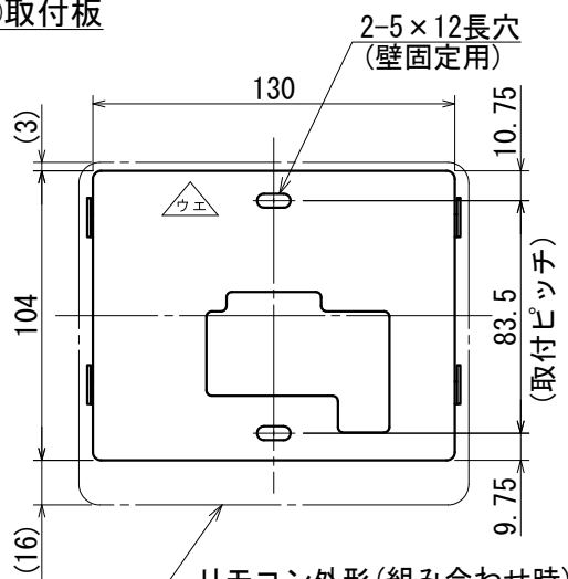
正面図
