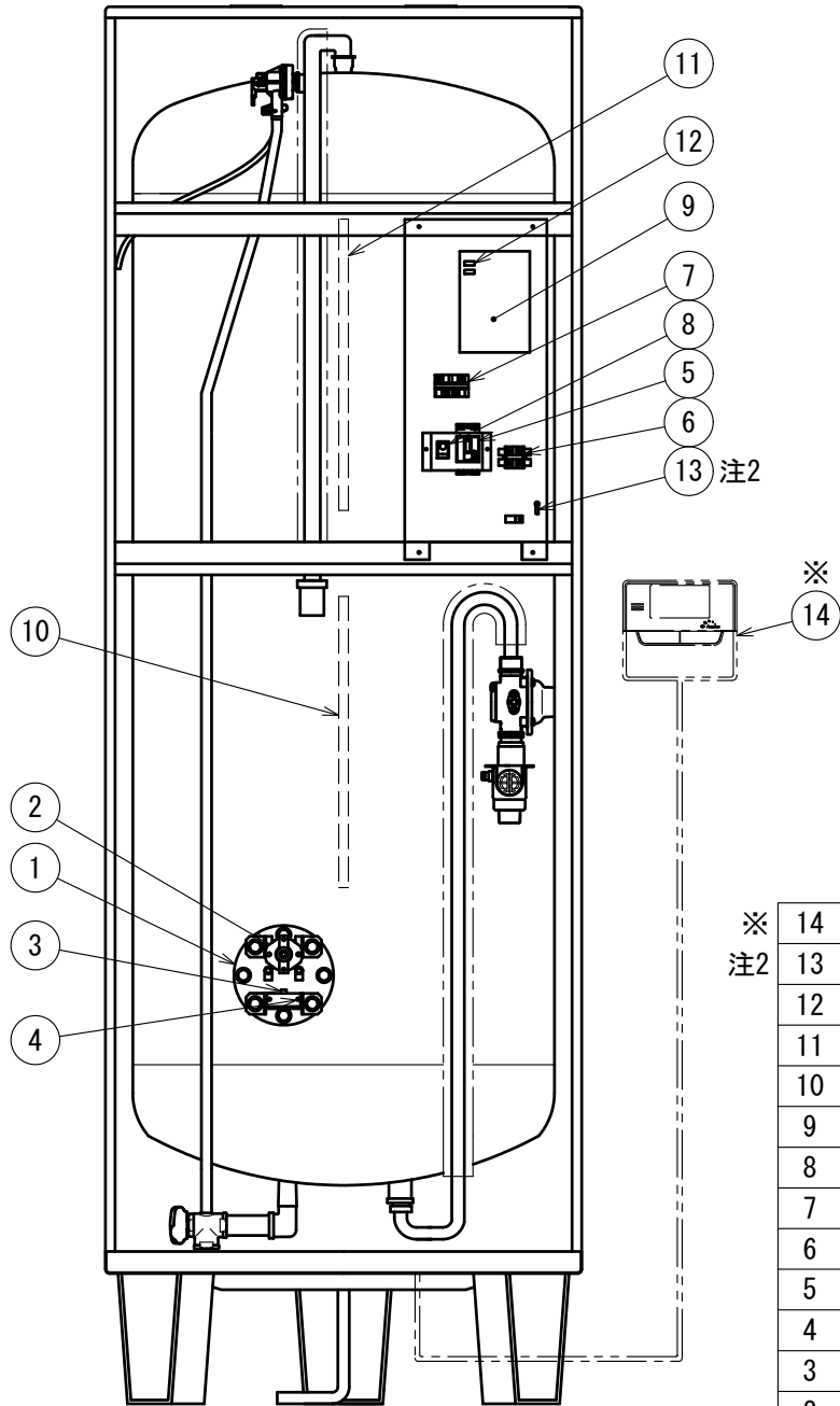
部品配置図
