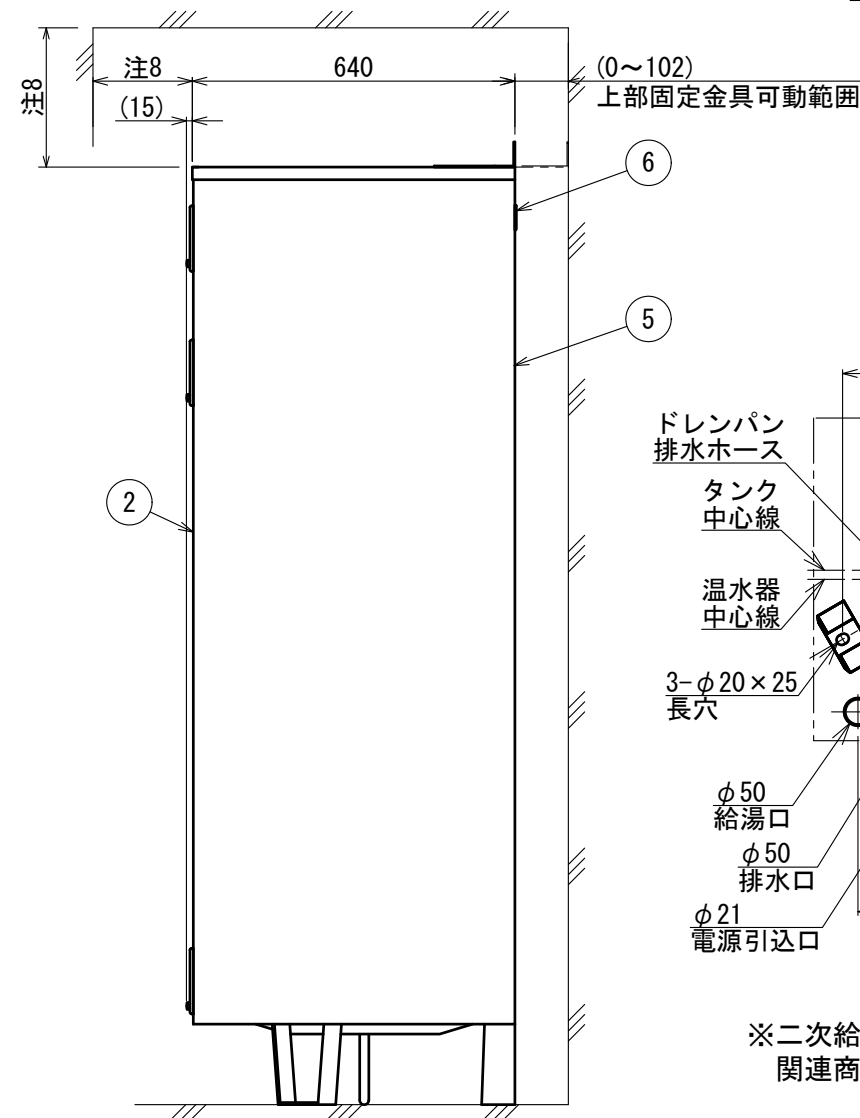
右側面図
