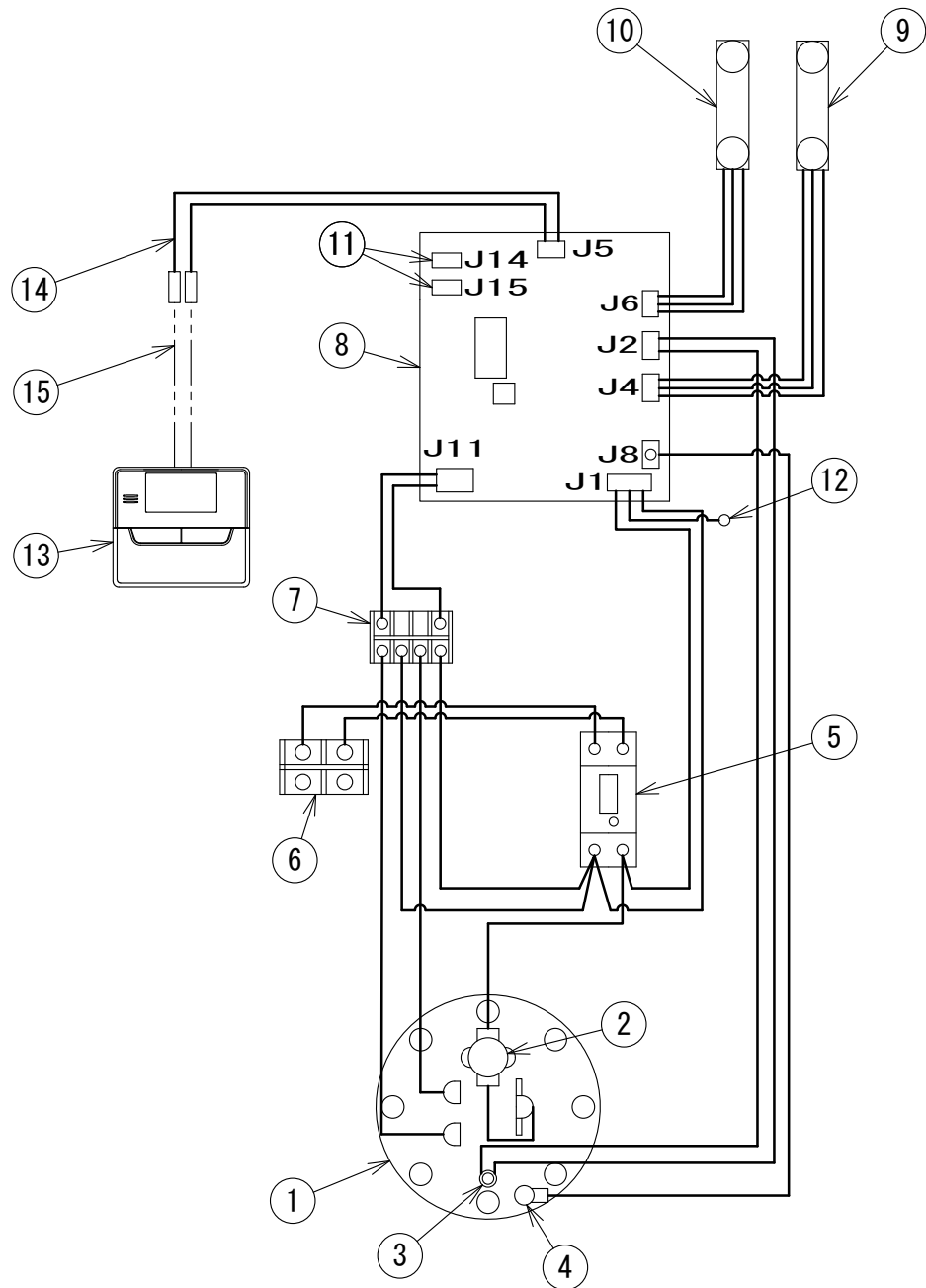
配線図
