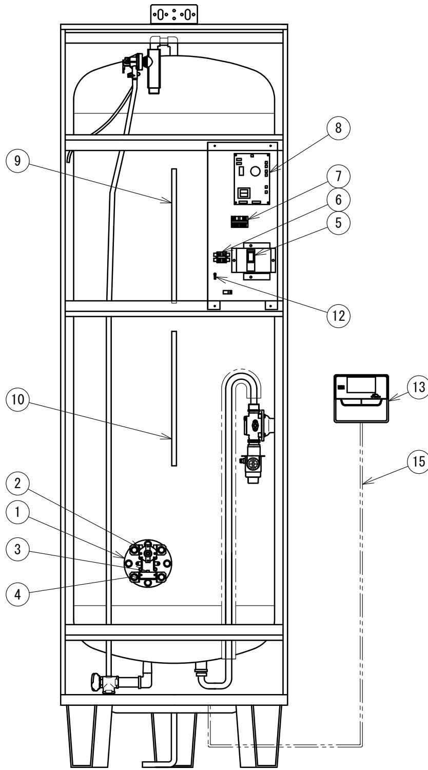
部品配置図
