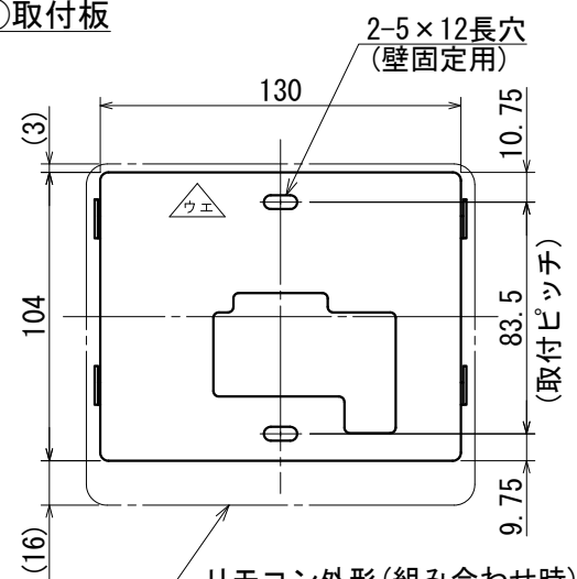
正面図
