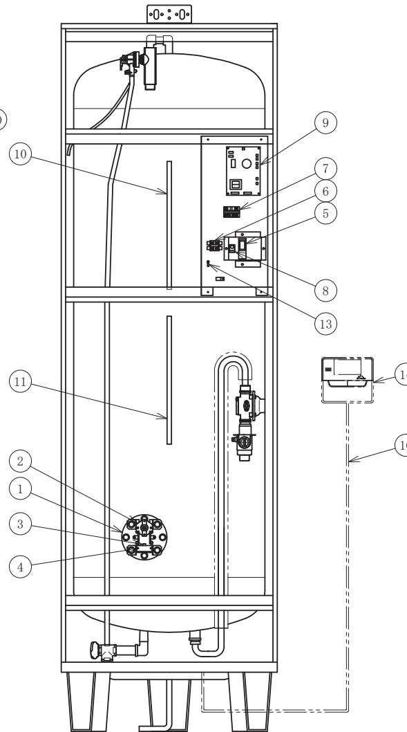
部品配置図
