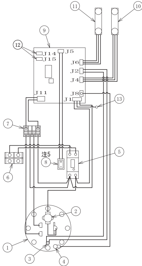
配線図
