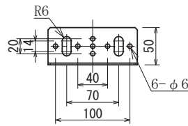
上部固定金具詳細
