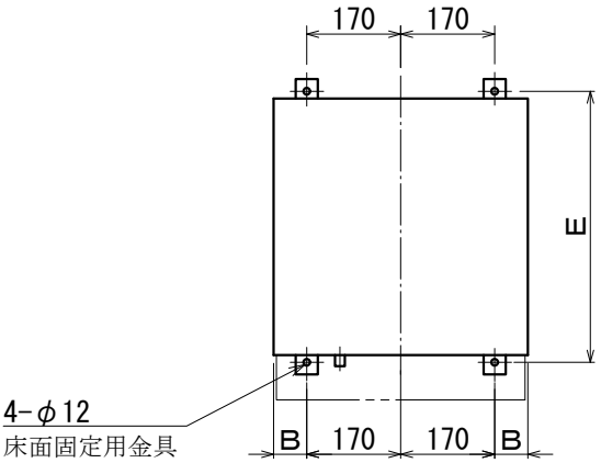
排水パン
