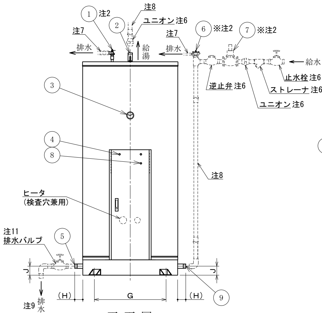
正面図
