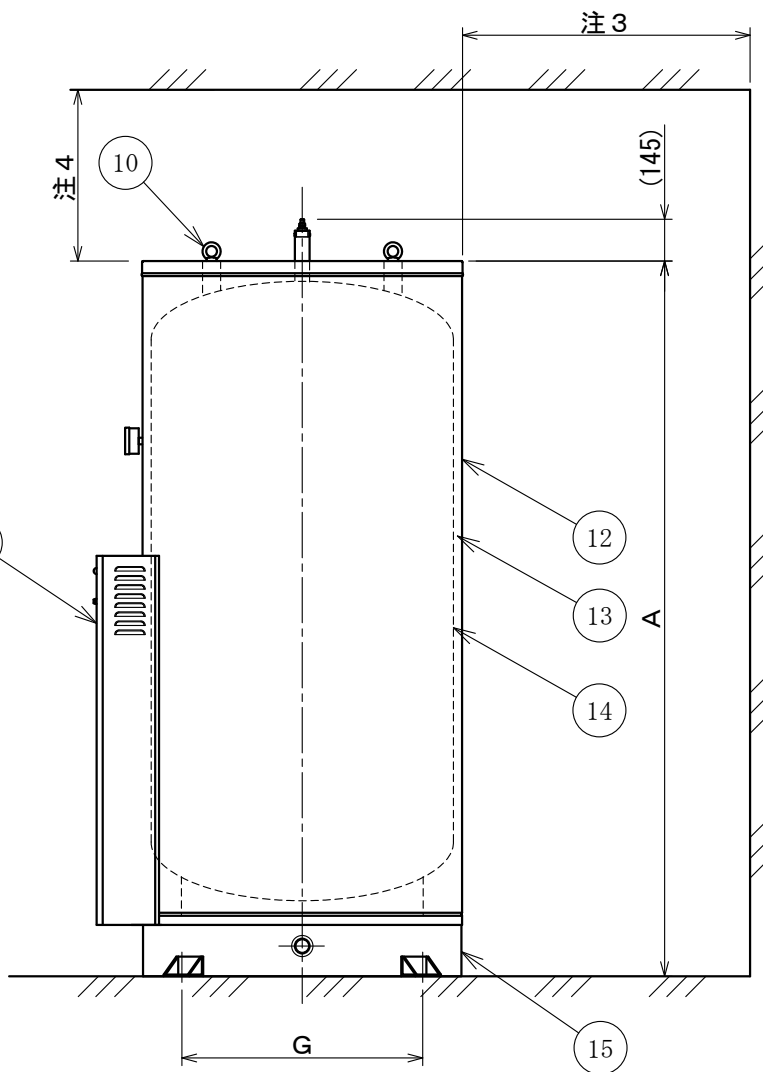
右側面図
