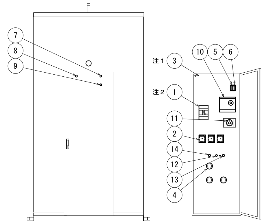
電装ケース部品配置図
