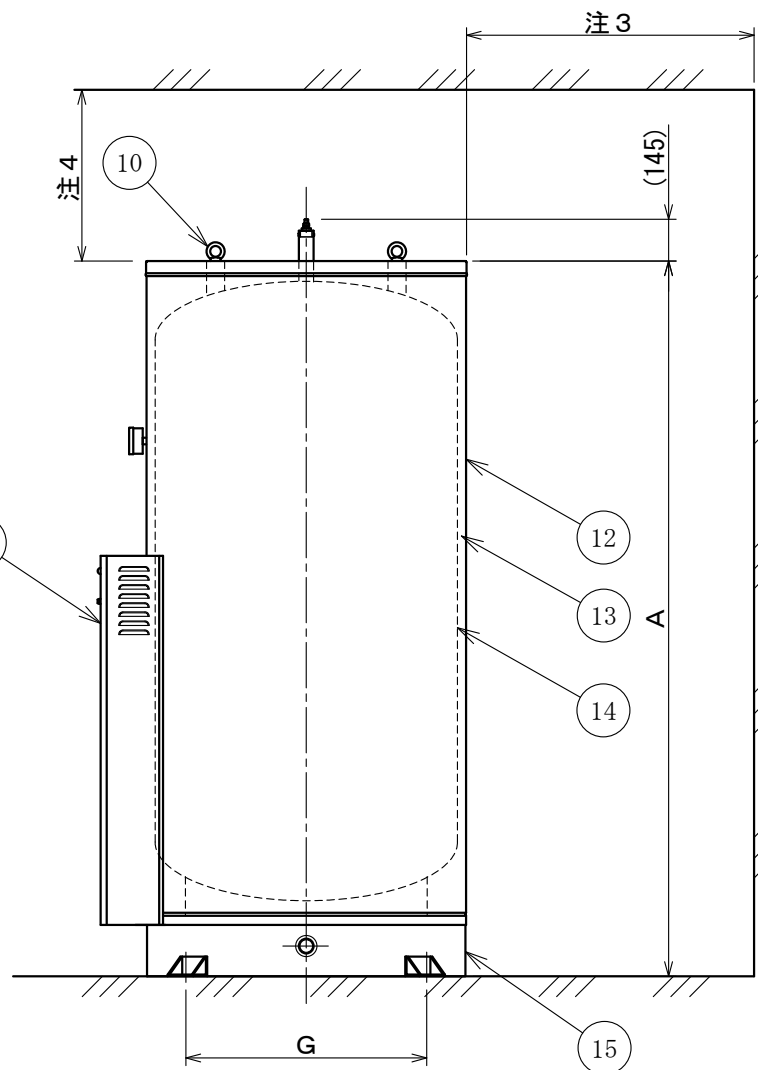
右側面図
