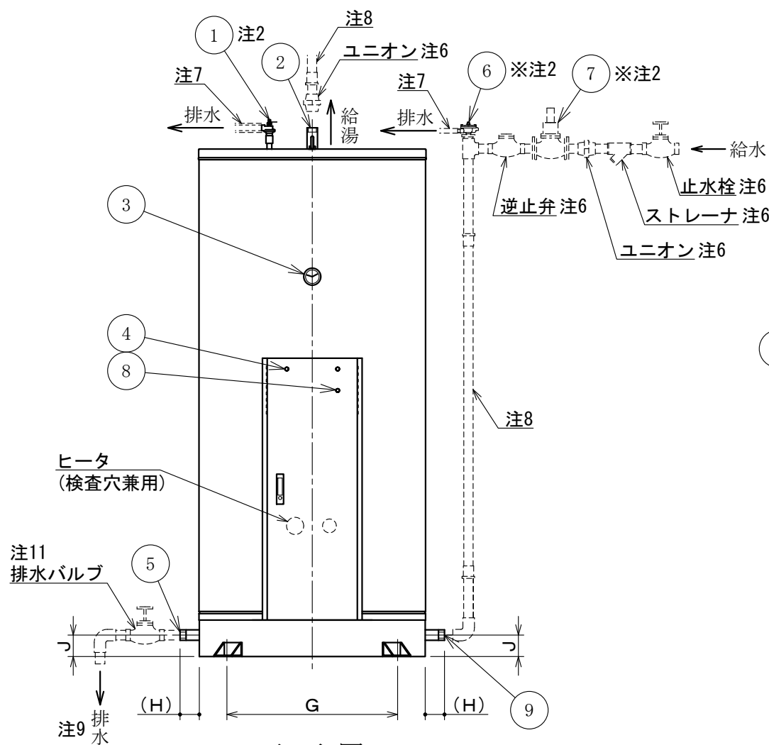
正面図
