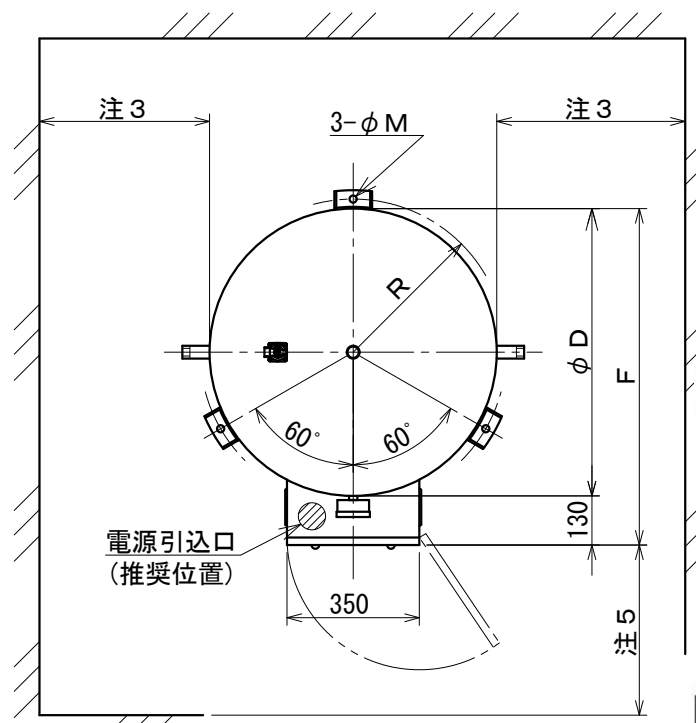
平面図
