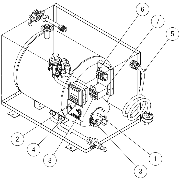
部品配置図
