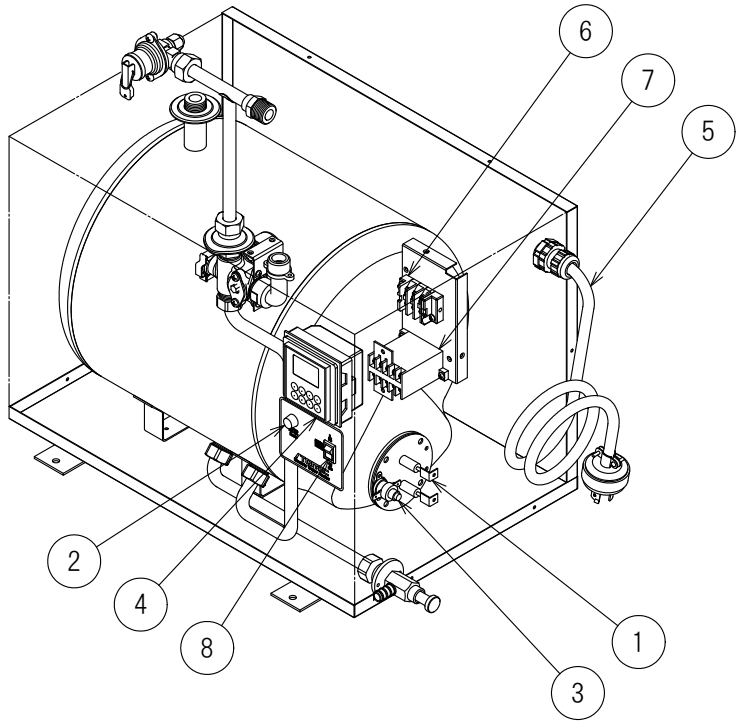
部品配置図
