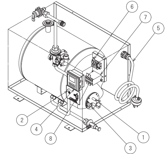
部品配置図
