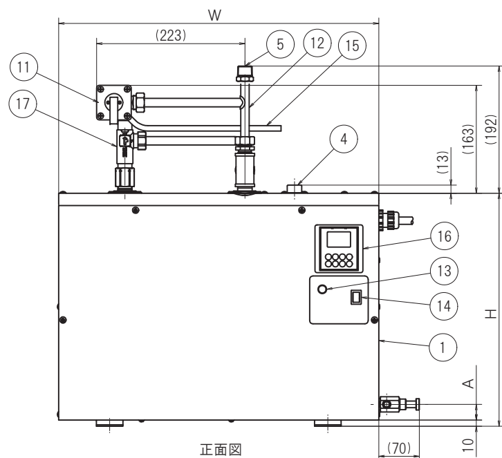
正面図
