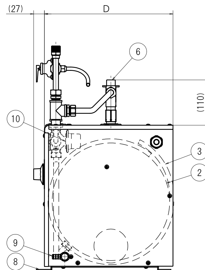
右側面図
