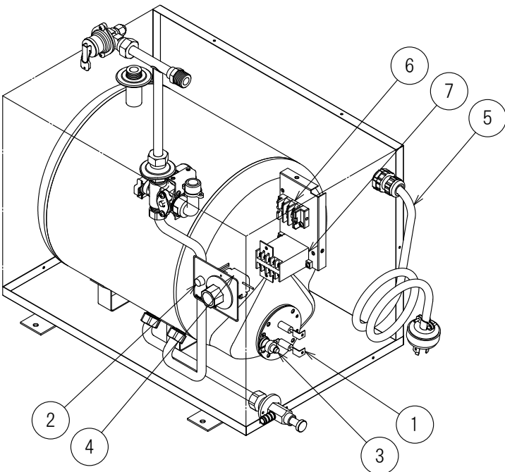
部品配置図
