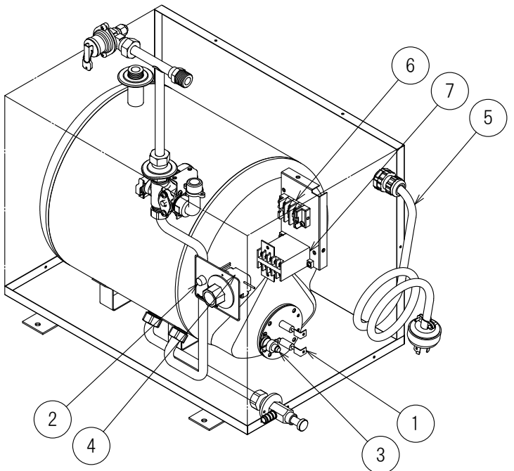
部品配置図
