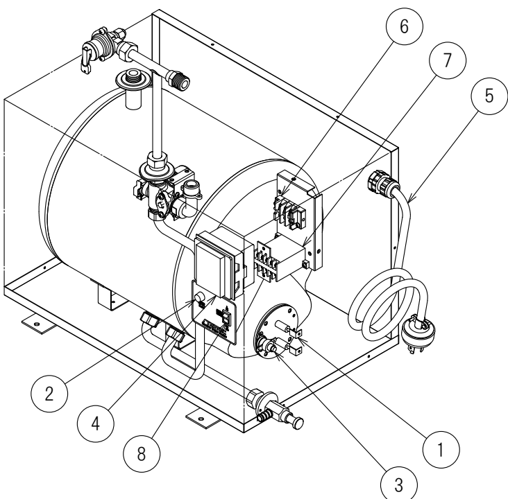
部品配置図
