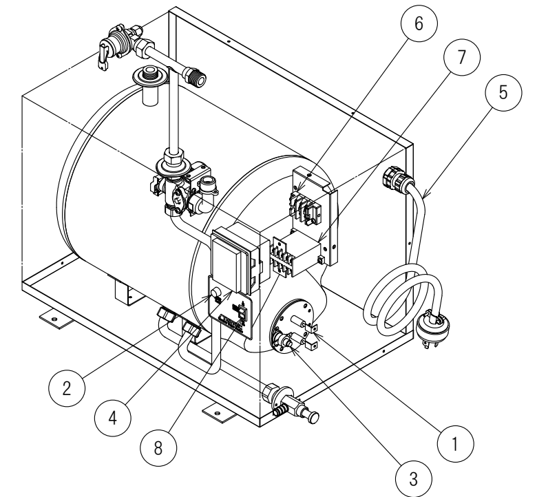
部品配置図
